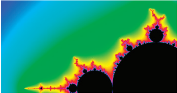
Conjunto de Mandelbrot
